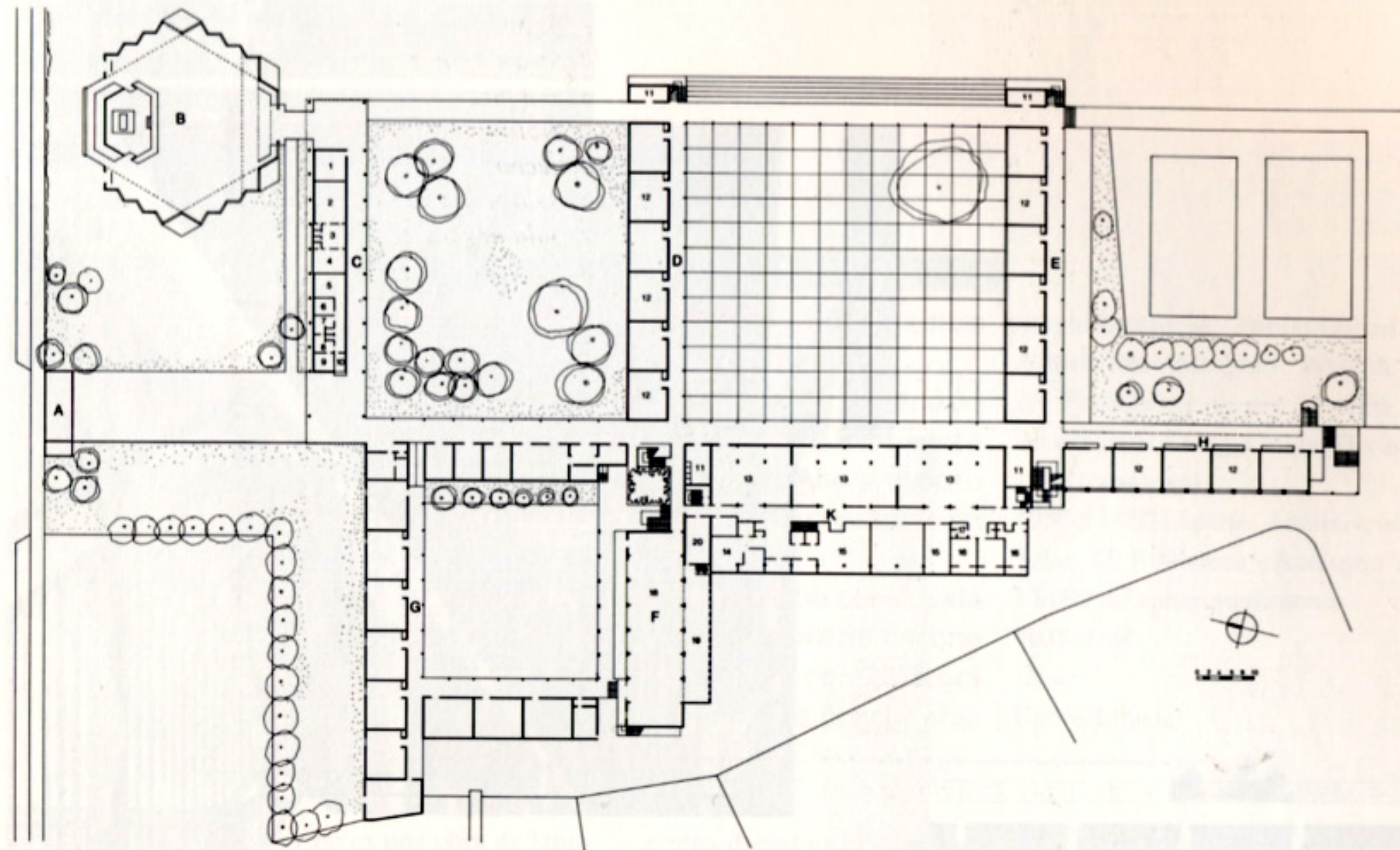
Planta general
