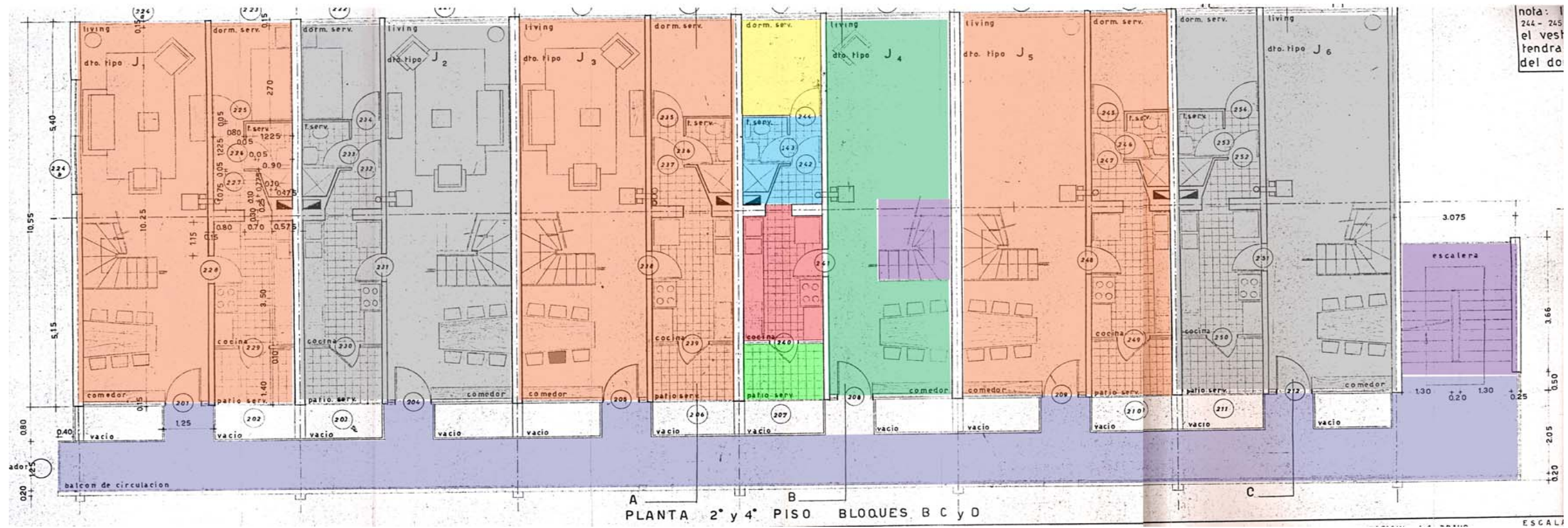
PLANTA PISOS 2 Y 4 TIPO DUPLEX.
