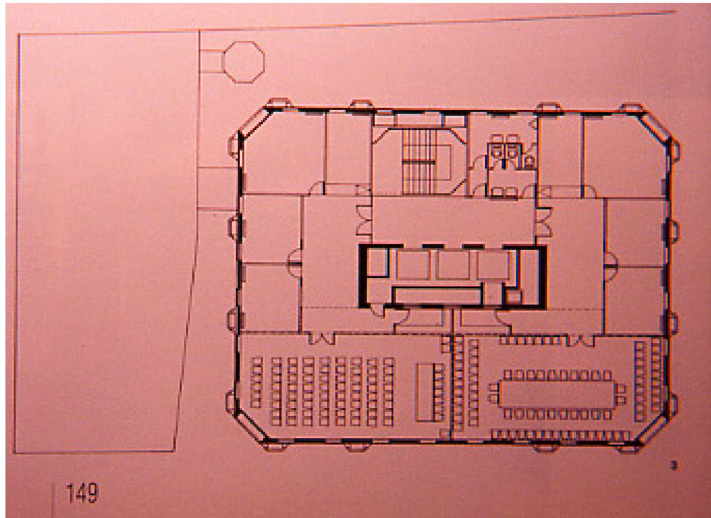
1 Planta tipo, en donde se lleva a la estructura a la periferia del edificio, para poder liberar el interior de estructura de pilares, manteniendo el núcleo rígido.
