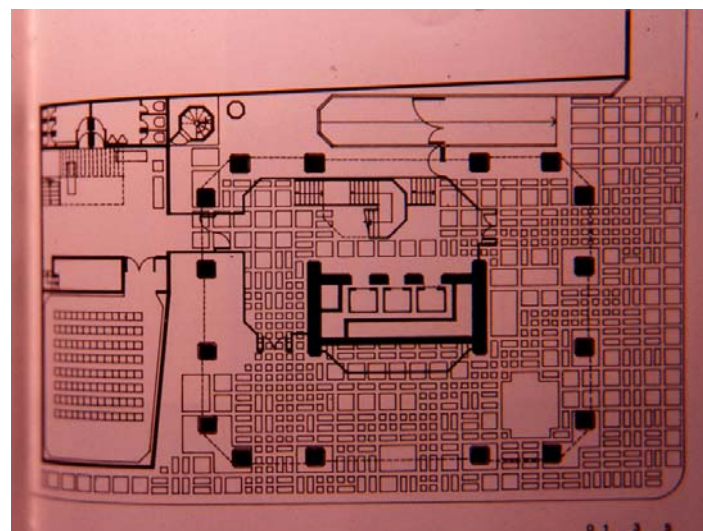
2 Planta de emplazamiento en donde se muestra la estructura perimetral y el núcleo rígido.
